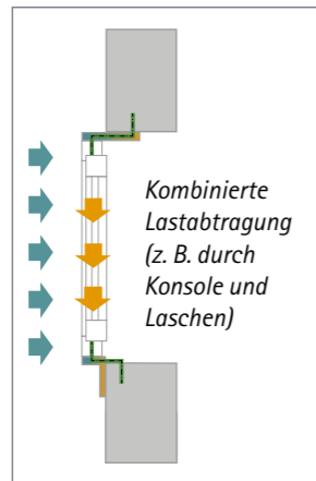
Einbaulage vor der Tragkonstruktion
