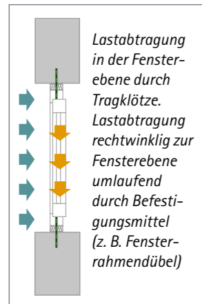
Einbaulage in der Leibung der Tragkonstruktion
