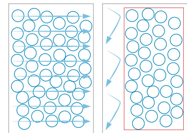
Vergleich ungeschützter und geschützter Dämmstoff: Rechts sind keine Luftbewegungen in der Porenstruktur möglich. Volle Dämmwirkung.
