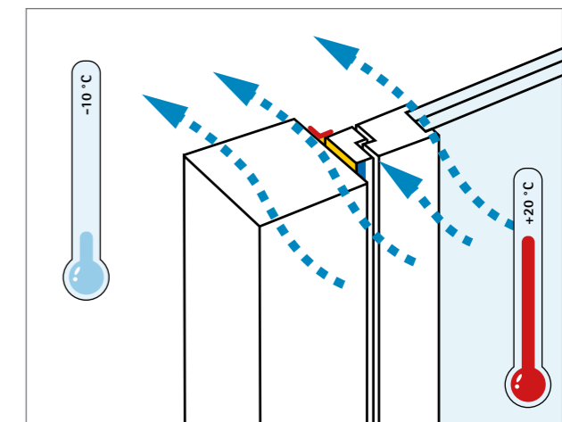
Diffusionsstrom im Winter: molekularer Feuchtetransport durch Bauteil und Fuge
